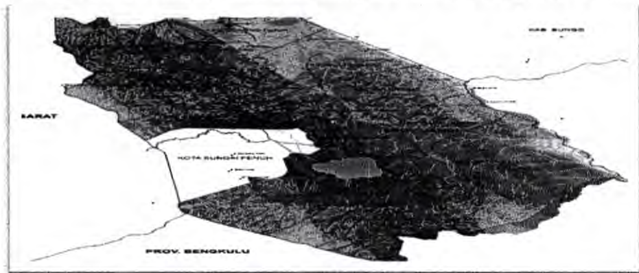
Gambar 2.3 Peta Kawasan Rawan Bencana Gempa Bumi di Kabupaten Kerinci
